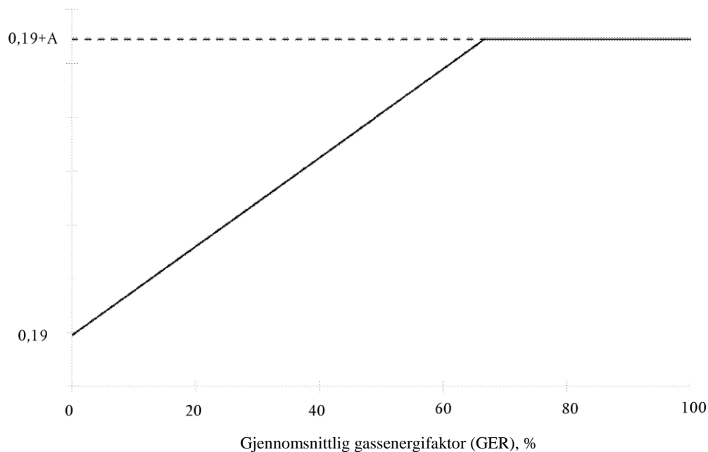
Figur 1. Diagram som viser grensen for utslipp av HC som funksjon av gjennomsnittlig GER
